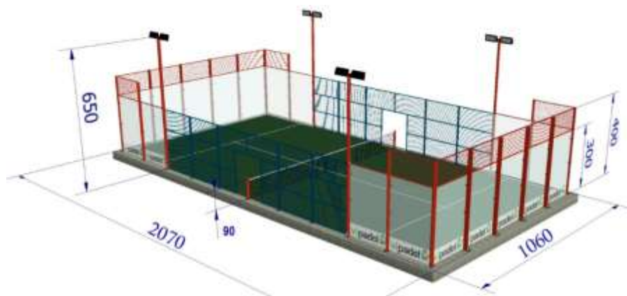
Figur 1- Illustration af padelbane
